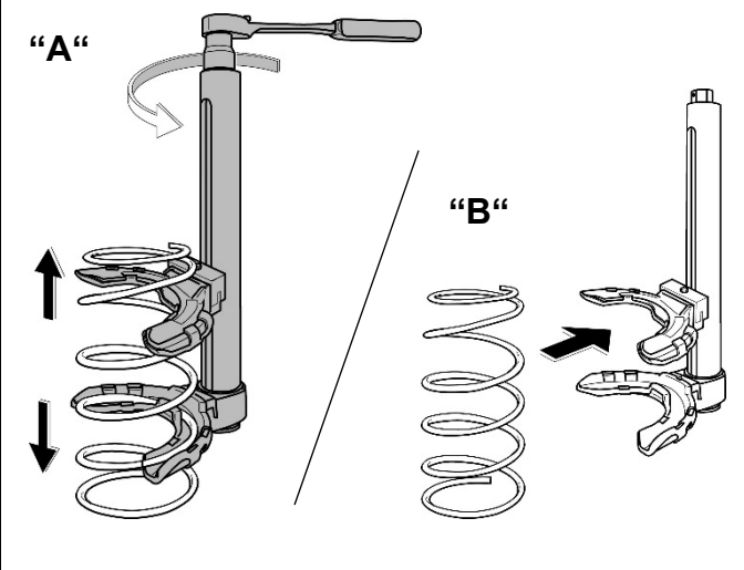
Fig. 15. Détendre le ressort.
