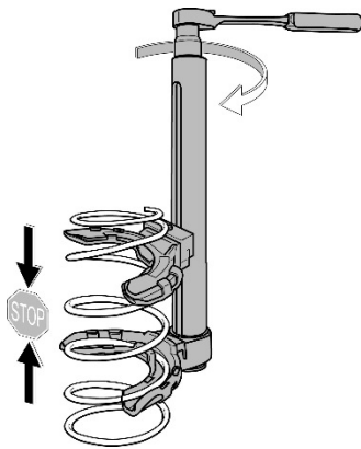
Fig. 26. Le ressort est comprimé.
