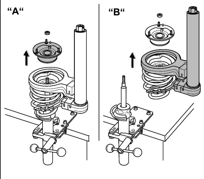
Fig. 20. Marquer les positions des coupelles.
