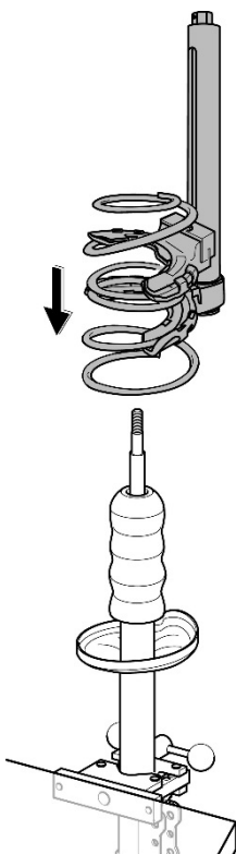
Fig. 27. Positionner le ressort sur la jambe de force/l'amortisseur.
