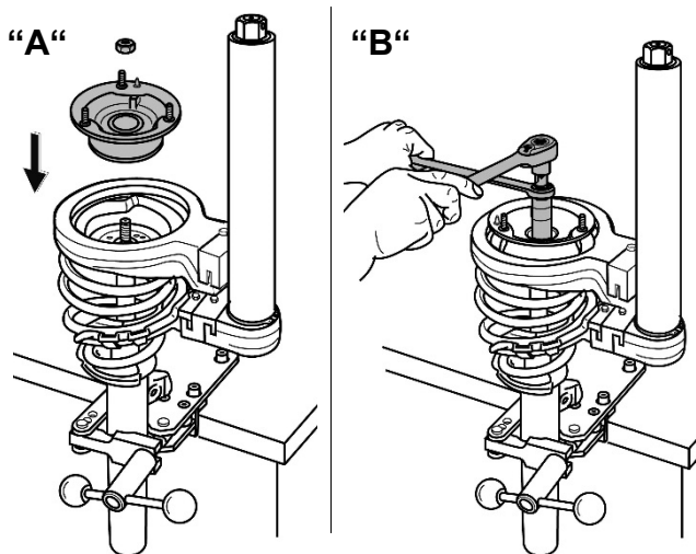
Fig. 37. Assembler la jambe de force.
