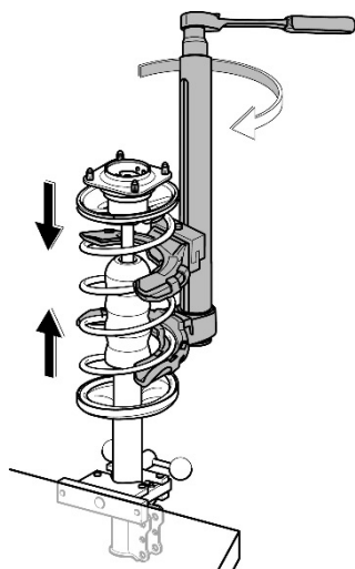
Fig. 12. Comprimer le ressort jusqu'à ce que l'écrou de tige de piston soit complètement relâché.
