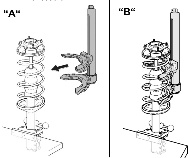
Fig. 11. Comprimer le ressort.
