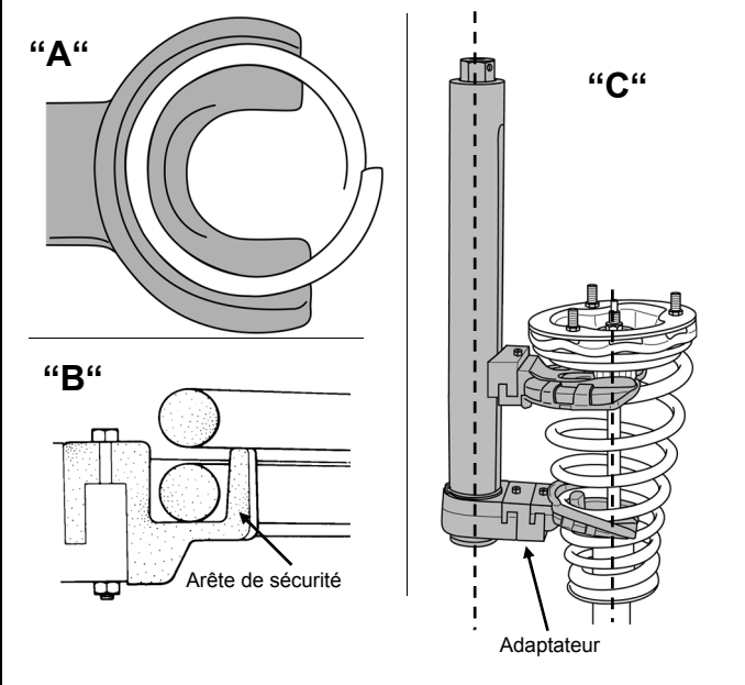
Fig. 5. Monter les coupelles sur le corps de compresseur (pour les ressorts standard).
